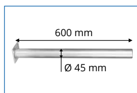
M1 Gaffel Varenr.: 8615003
