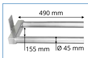
M2 Dobbelt gaffel Varenr.: 8615002
