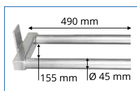
M2 Dobbelt gaffel Varenr.: 8615004
